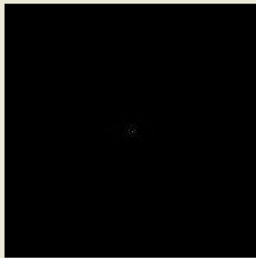
k-space
